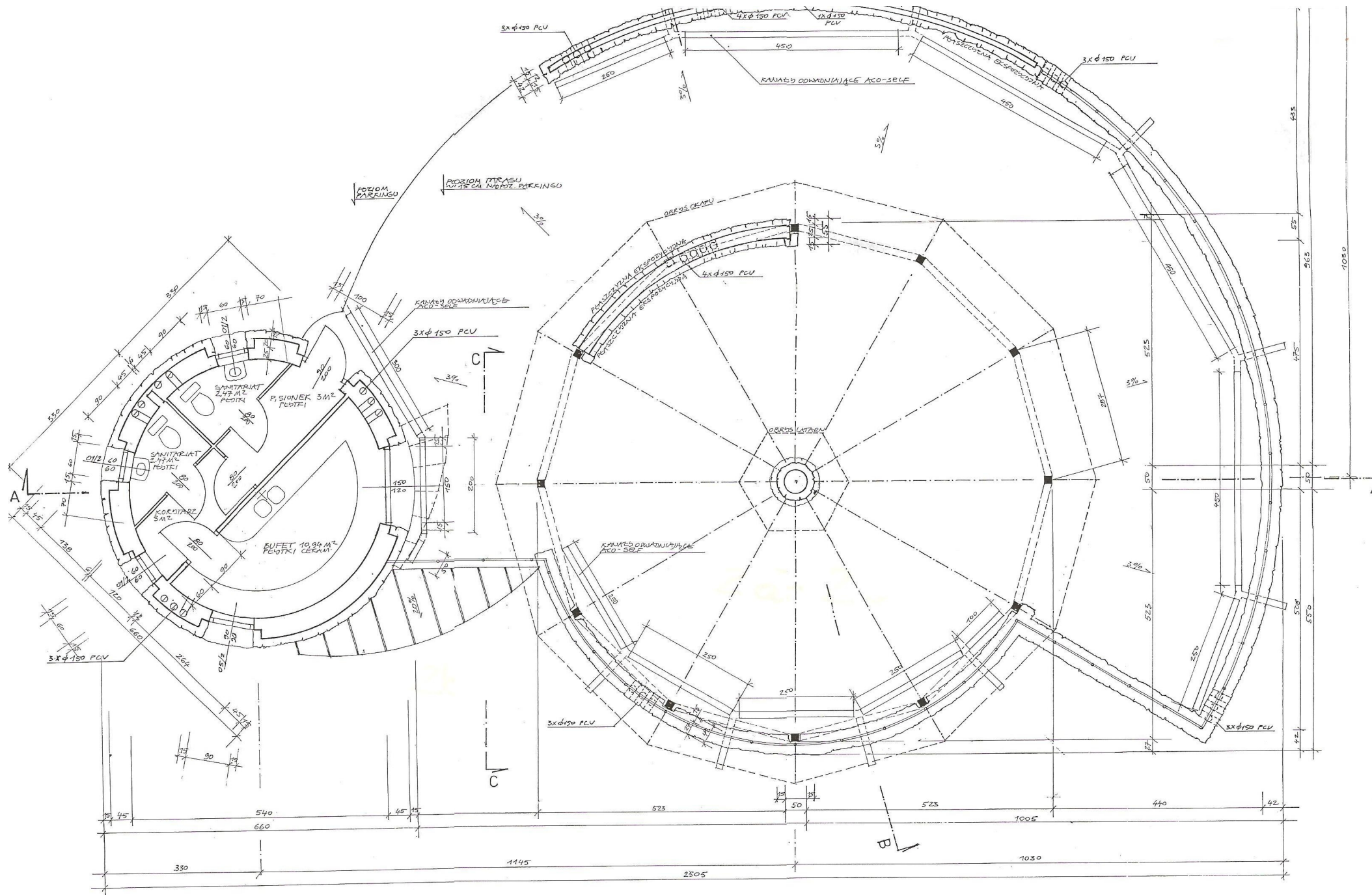
PAWILON EKSPOZYCYJNY W CZORSZTYNIE Rzut wysokiego parteru 1:50 rys.3 Autorzy: arch.A. Böhm arch.W.Kosiński
